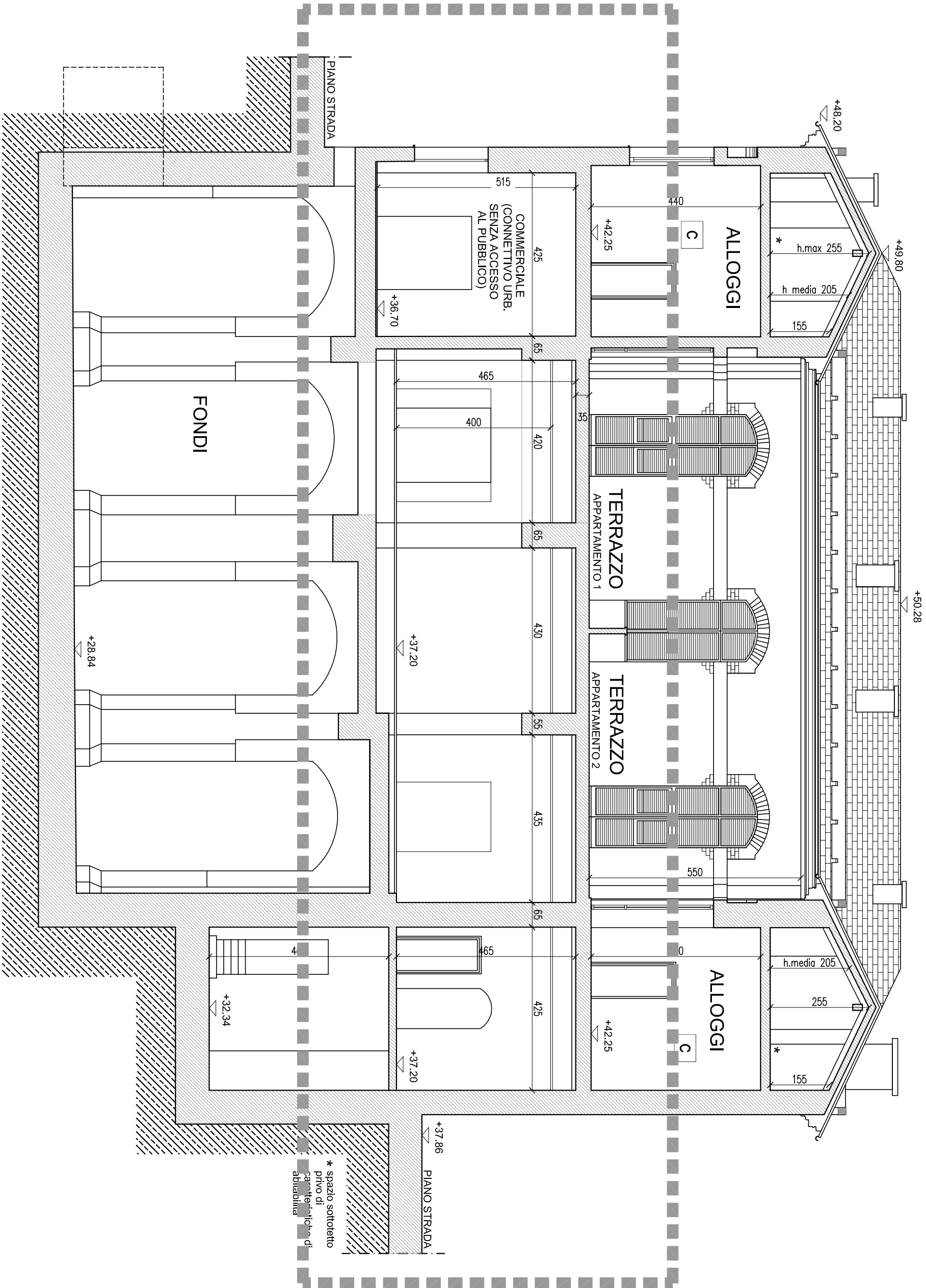
LONGITUDINALE B-B
