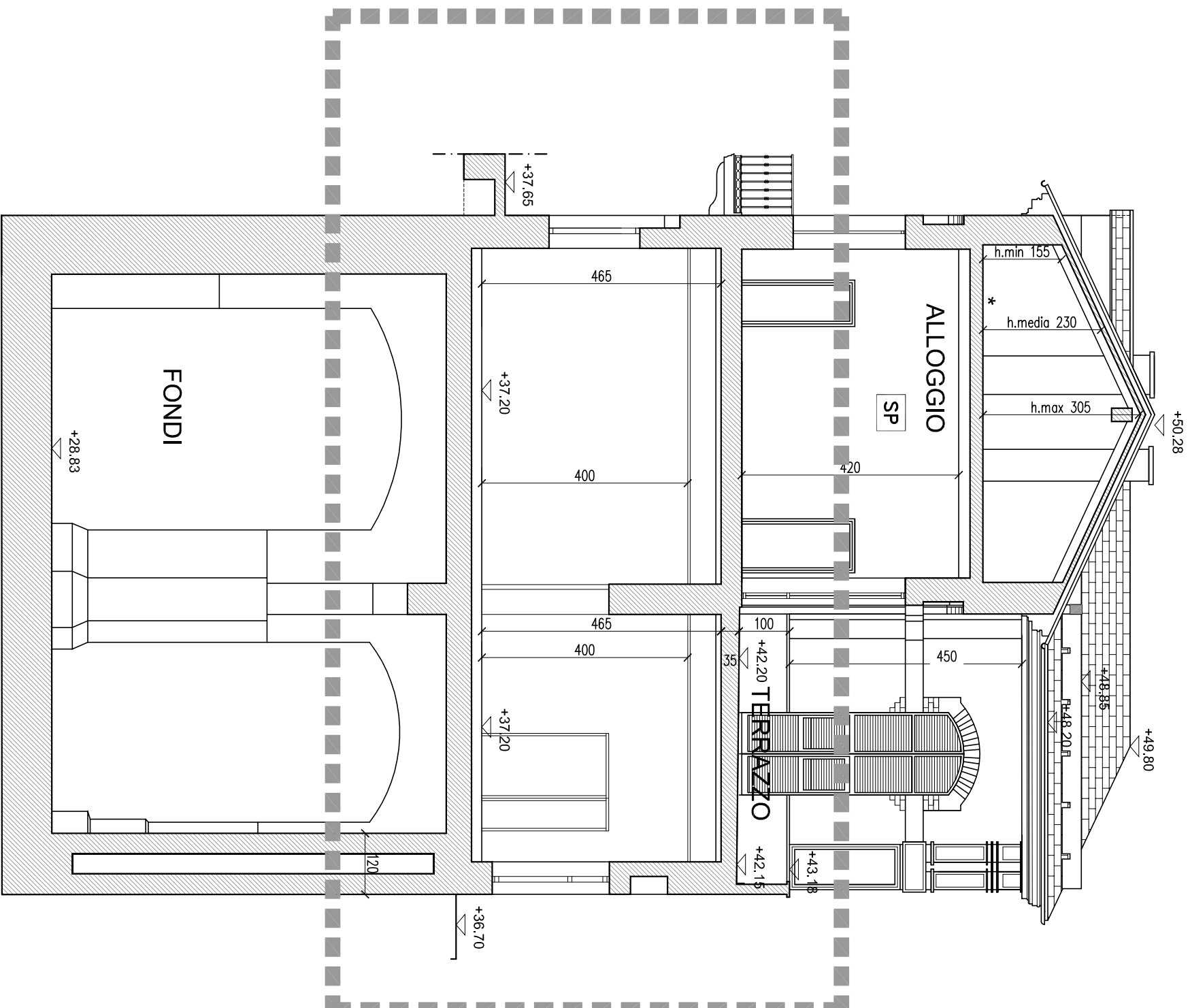
TRASVERSALE A-A
